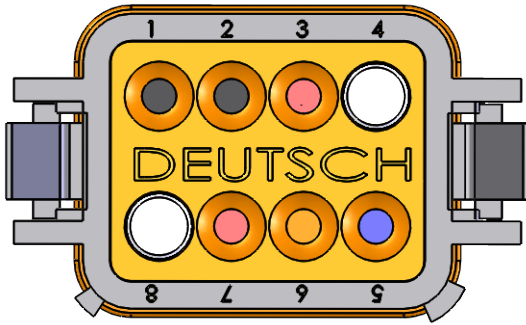
0857-1 Current Sense
